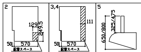
レイアウト展開図A
