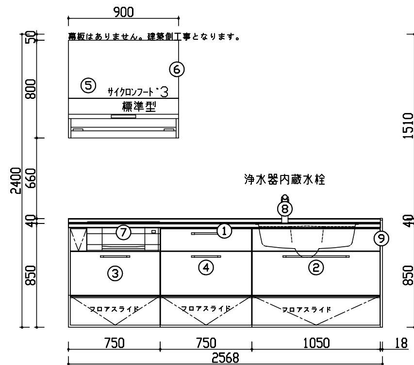
レイアウト展開図A
